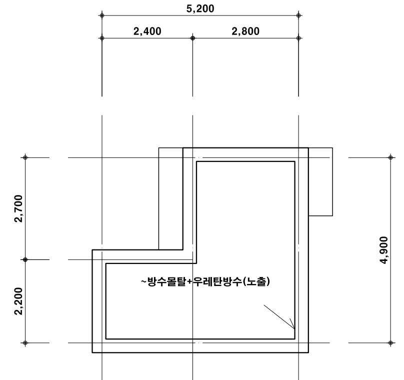
옥탑지붕 평면도
